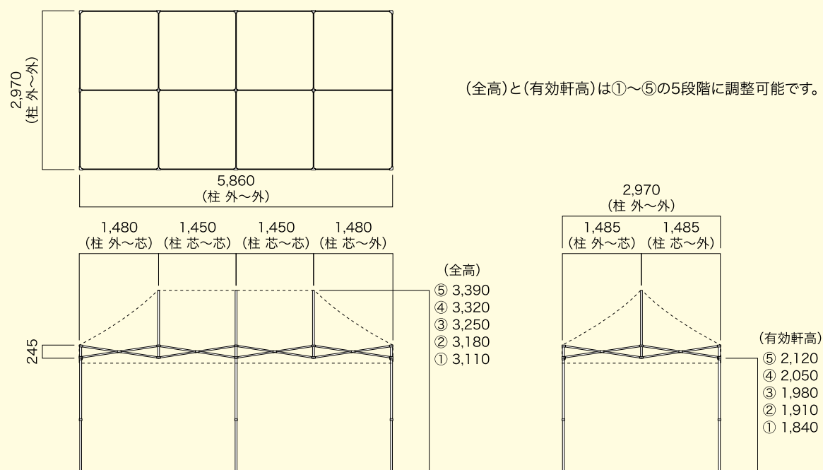
フレーム・天幕 詳細寸法 3m×6m
