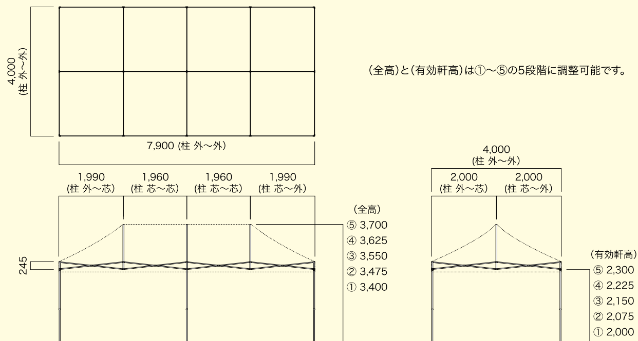
フレーム・天幕 詳細寸法 4m×8m
