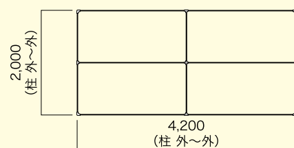
フレーム・天幕 詳細寸法 2m×4.2m
