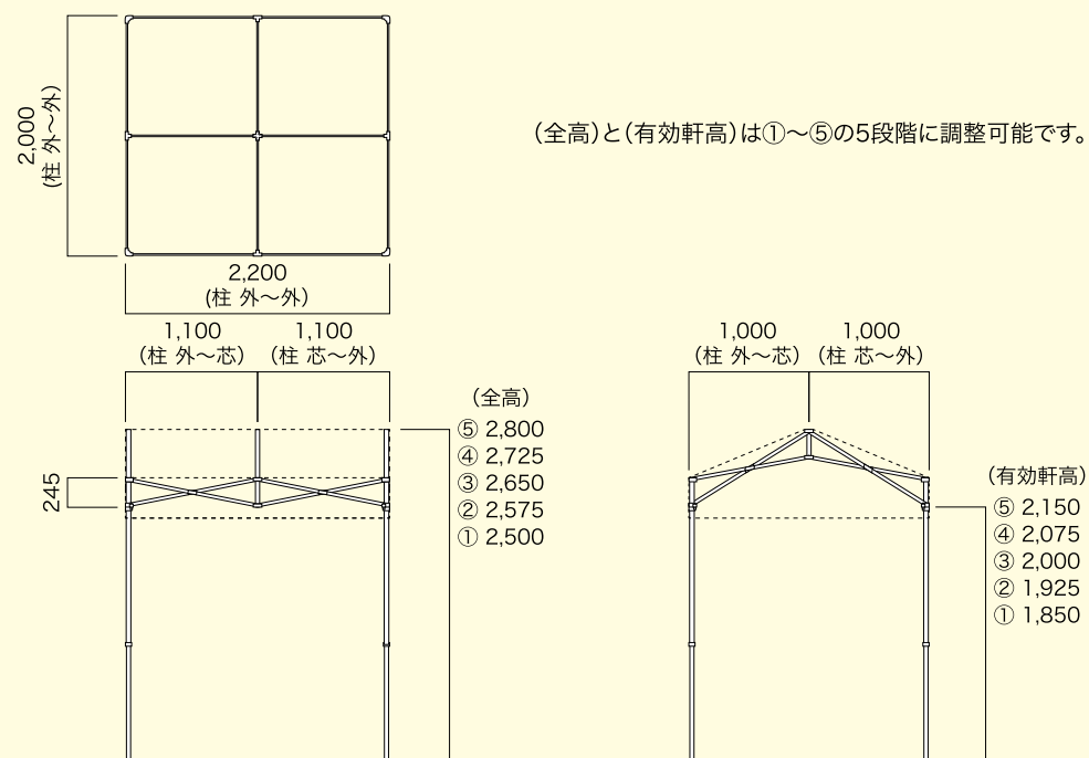
フレーム・天幕 詳細寸法 2m×2.2m
