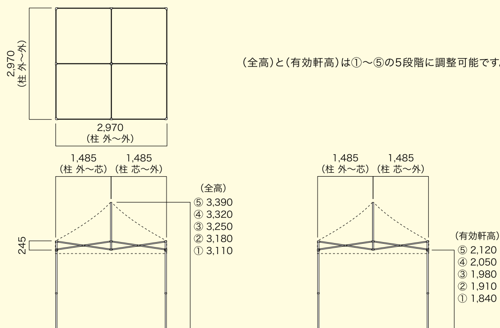
フレーム・天幕 詳細寸法 3m×3m
