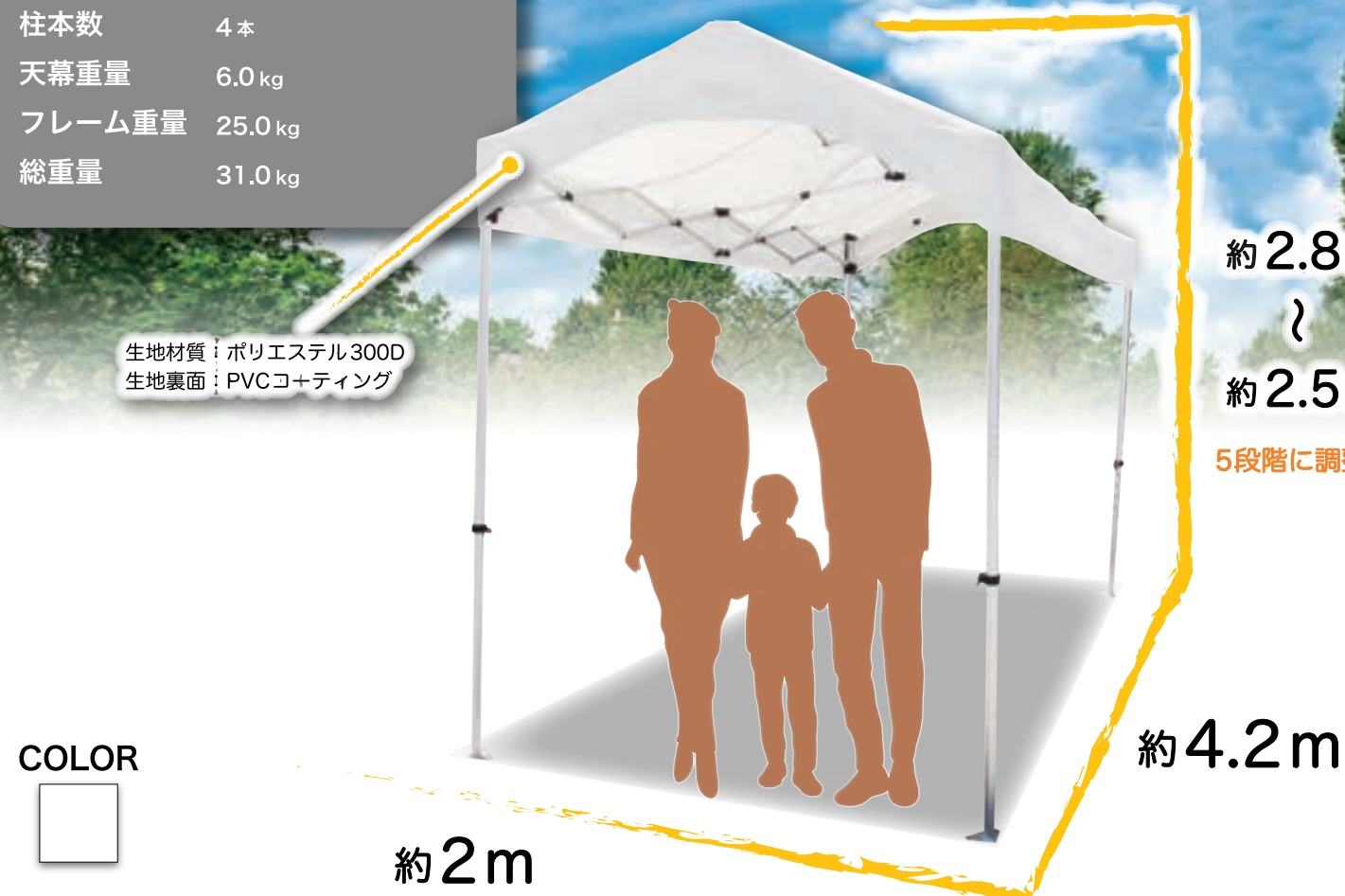
フレーム・天幕 詳細寸法 2m×4.2m
