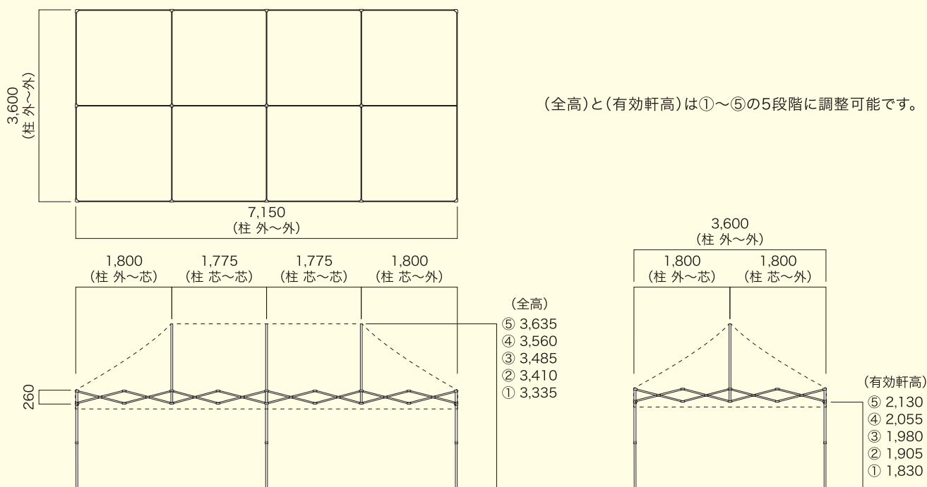
フレーム・天幕 詳細寸法 3.6m×7.2m
