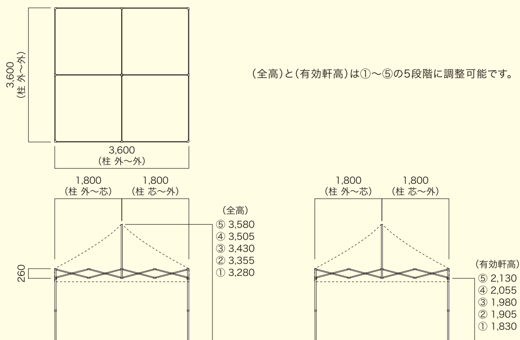
フレーム・天幕 詳細寸法 3.6m×3.6m
