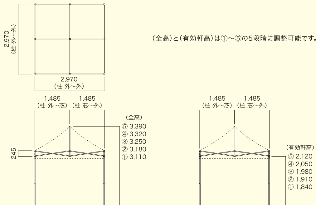
フレーム・天幕 詳細寸法 3m×3m
