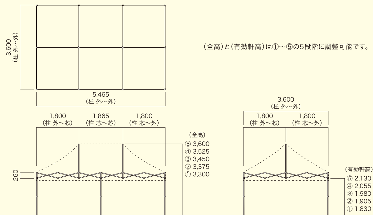
フレーム・天幕 詳細寸法 3.6m×5.4m
