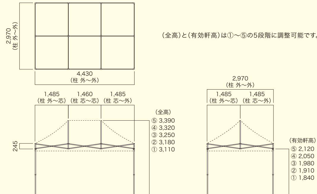
フレーム・天幕 詳細寸法 3m×4.5m
