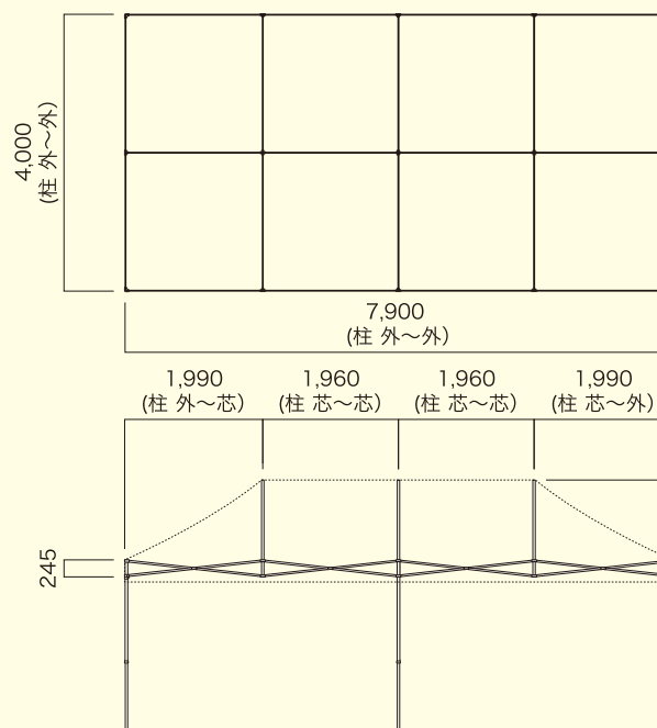
フレーム・天幕 詳細寸法 4m×8m
