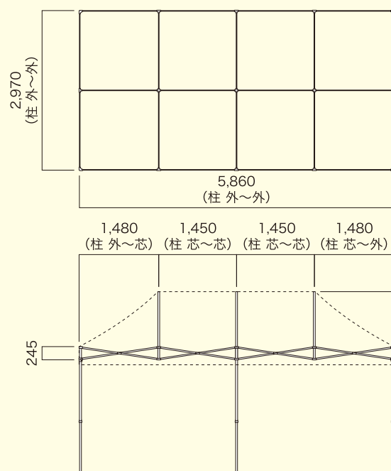
フレーム・天幕 詳細寸法 3m×6m
